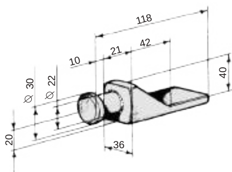
15001170 Piantone centrale kg 0,400
