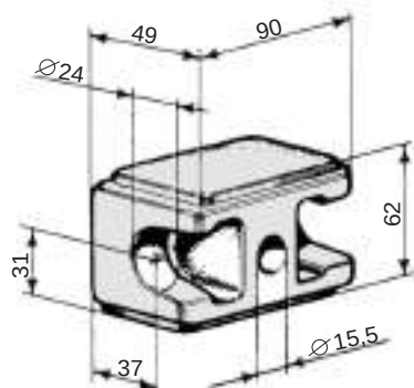
15001130 Blocco centrale kg 1,170
