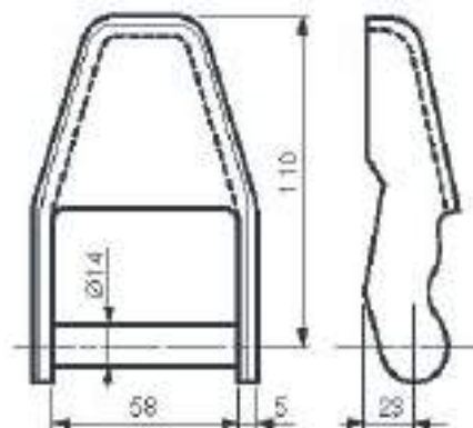
15000440 Supporto barra kg 0,355
