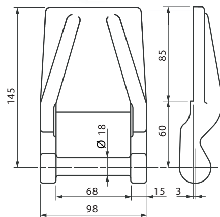
15000520 Cerniera sponda kg 0,920
