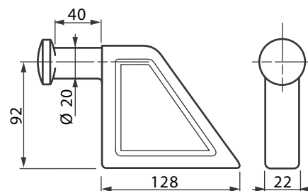
15001550 Piantoncino kg 0,400
