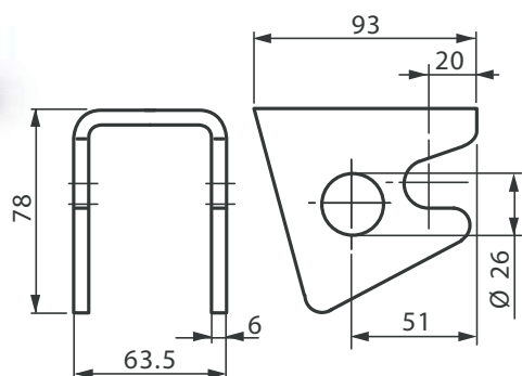
15000580 Supporto barra kg 0,635
