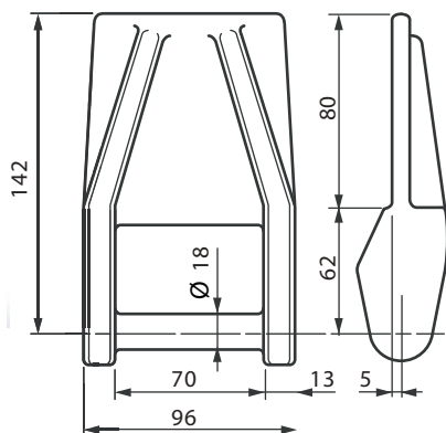
15000550 Supporto barra kg 0,550
