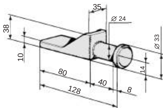
15001160 Piantone posteriore kg 0,550
