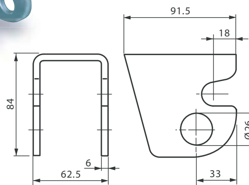
15000540 Paletta kg 0,730
