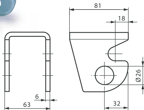
15000530 Paletta kg 0,600
