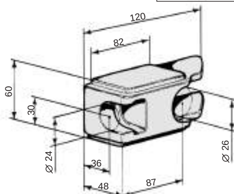
15001180 Blocco posteriore kg 1,400
