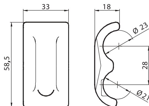
20010930 Paletta kg 0,220
