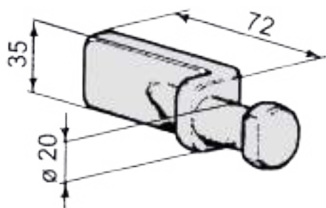
15001510 Piantone kg 0,370
