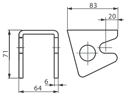
15000580 Supporto barra kg 0,635
