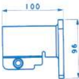
40058820 Supporto in plastica per tubo Ø 42
