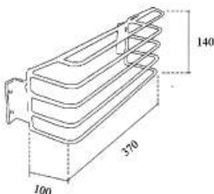
40050880 Griglia universale tipo ASTRA 370 x 140 x 100 mm
