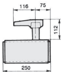
35042070 Supporto per gamba sinistro - kg 8,100
