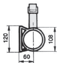
35042060 Supporto per gamba destro - kg 8,100
