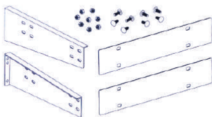
Fissaggio orizzontale
