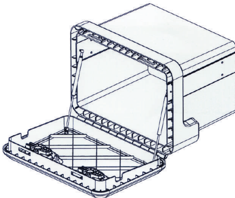
Fissaggio orizzontale
