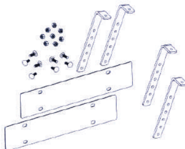
Fissaggio verticale
