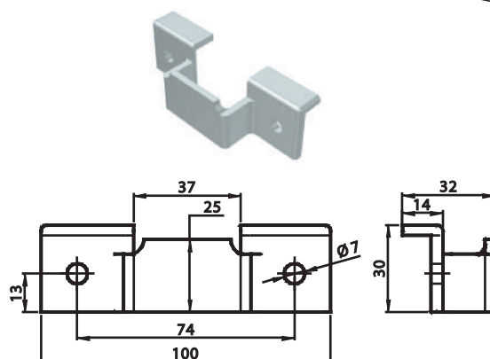
20011100 Riscontro zincato kg 0,100
