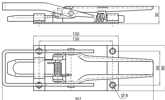
20011090 Serratura a tirante kg 0,970
