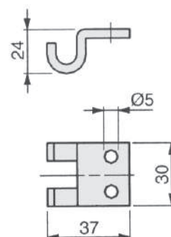
20011380 Riscontro zincato per chiusura kg 0,036
