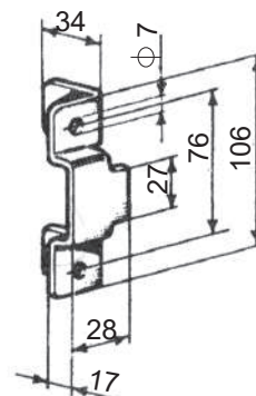
20011080 Riscontro zincato kg 0,300
