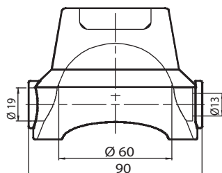
25020080 Supporto sfera Ø 60 con asola - kg 1,200
