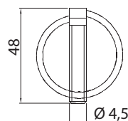
25020090 Copiglia zincata a scatto Ø 4,5 kg 0,025
