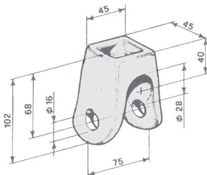
25020900 Supporto per ribaltabili agricoli kg 0,900
