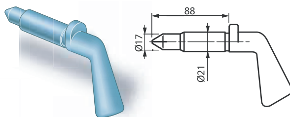
25020690 Spinotto fori differenziati kg 0.430
