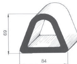
65100540 Paracolpo posteriore in gomma nera EPDM, tagli m 2,6
