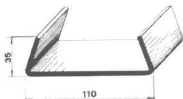
65100510 Profilo di fissaggio in acciaio zincato barre m 2,6
