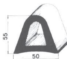
65100520 Paracolpo posteriore in gomma nera EPDM, tagli m 2,2
