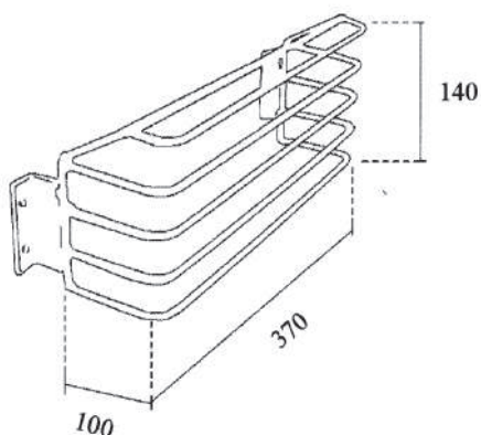
40050880 Griglia universale tipo ASTRA 370 x 140 x 100 mm
